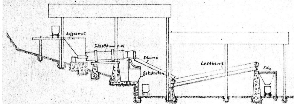
Schwerspataufbereitungsanlage der Schwerspatgrube Ohlsbach GmbH. M = 1:100
