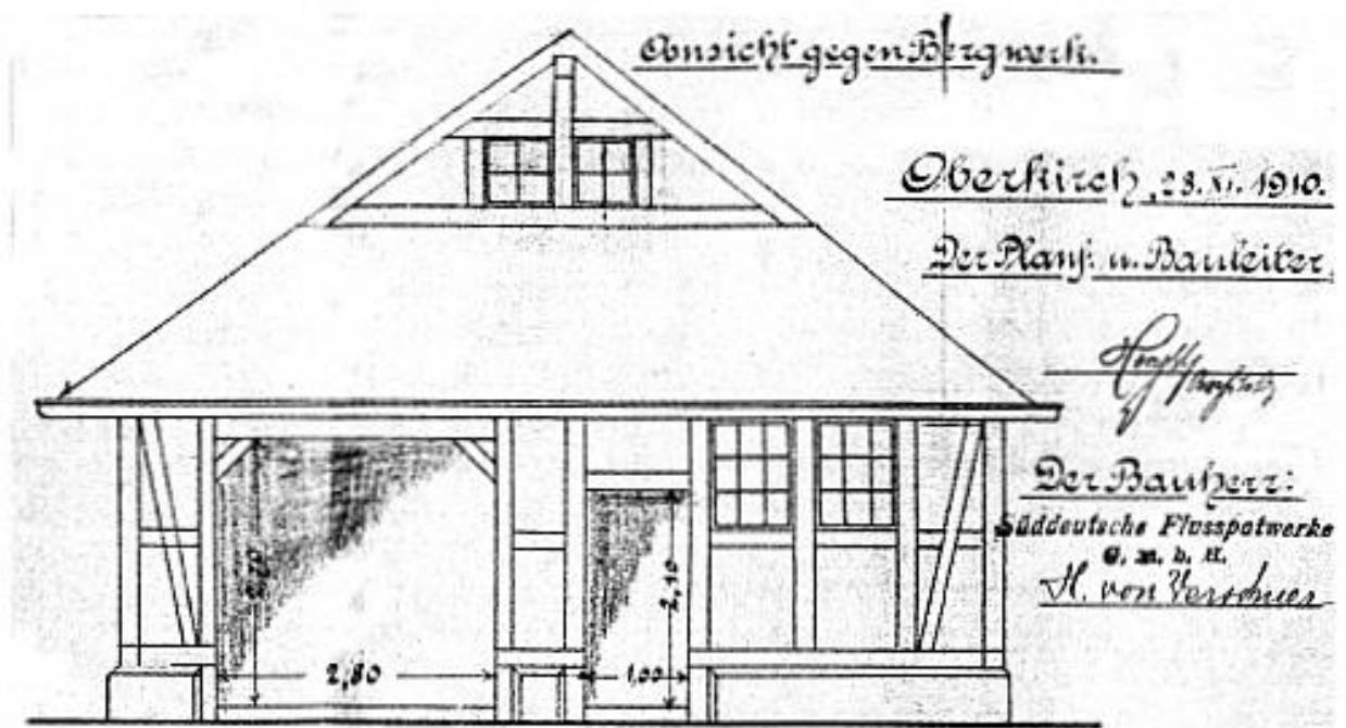
Planzeichnung der von den Süddeutschen Flußspatwerken im Jahre 1911 neu errichteten Kaue der Grube Hesselbach.
