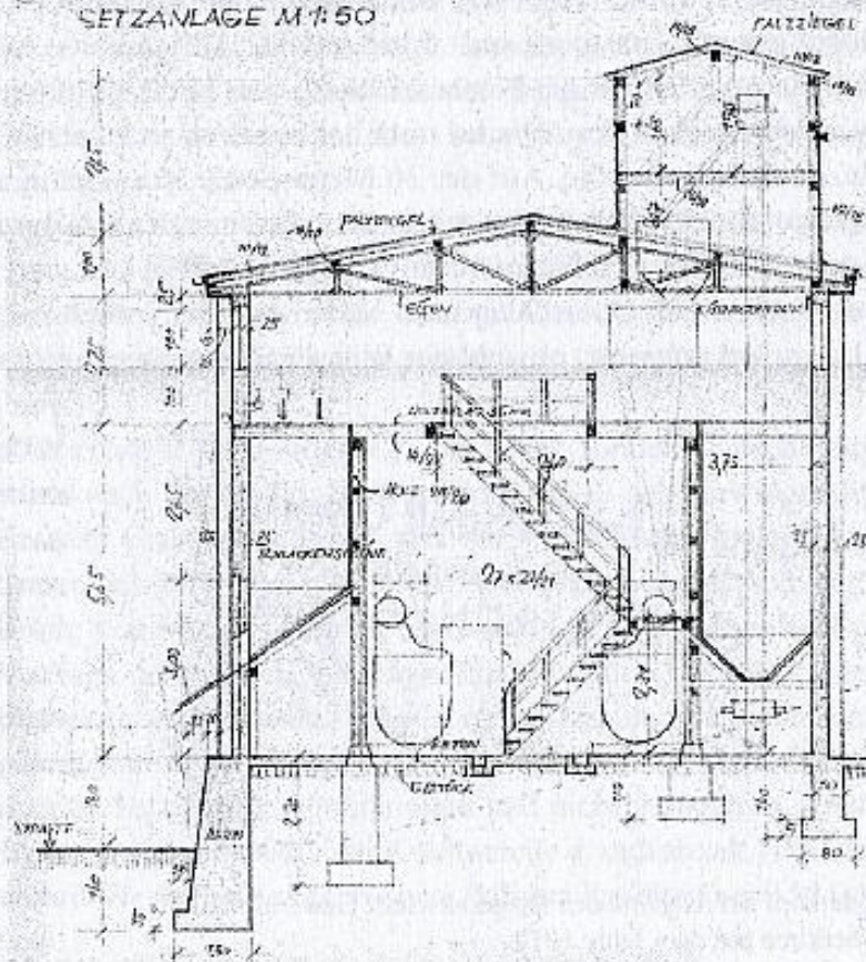
SPATWERK HESSELBACH SETZANLAGE M 1:50
