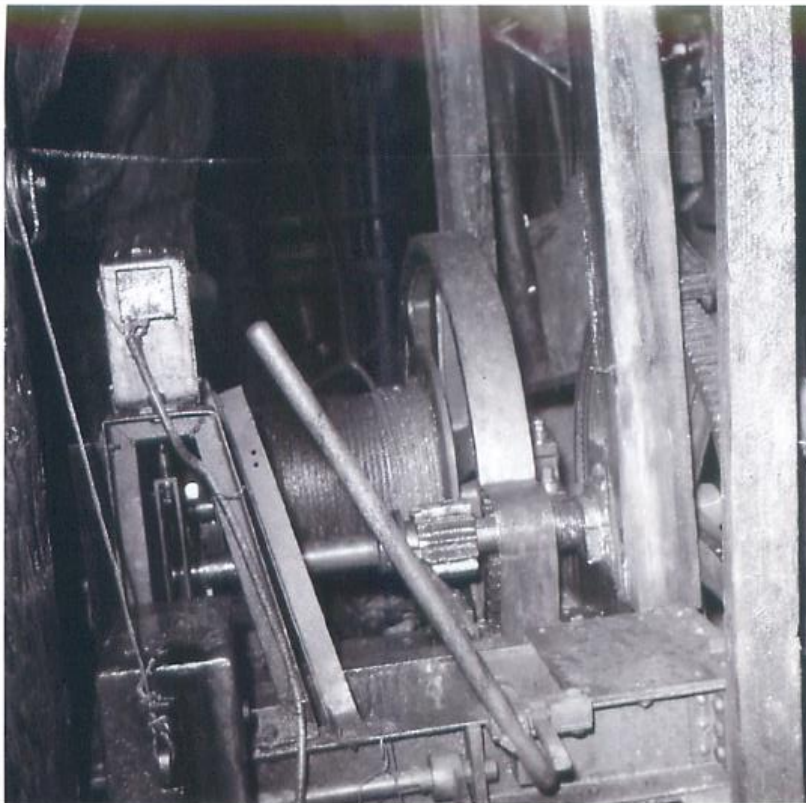
Förderhaspel zwischen 1. und 2. Sohle
