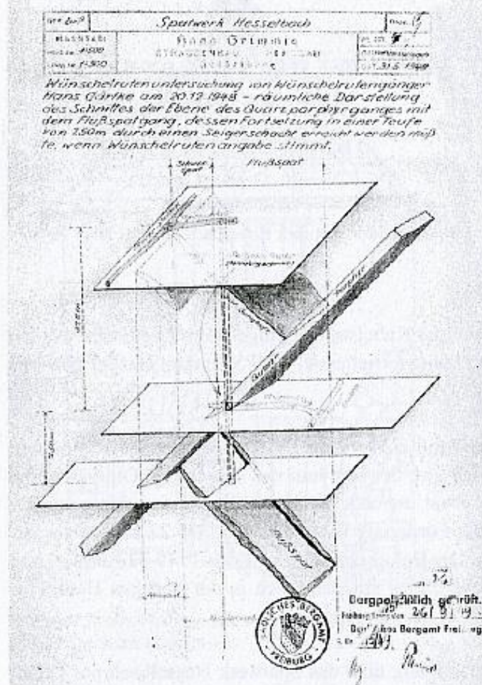
Räumliche Darstellung des mit Hilfe der Wünschelrute vorhergesagten Gangverlaufs (1949).
