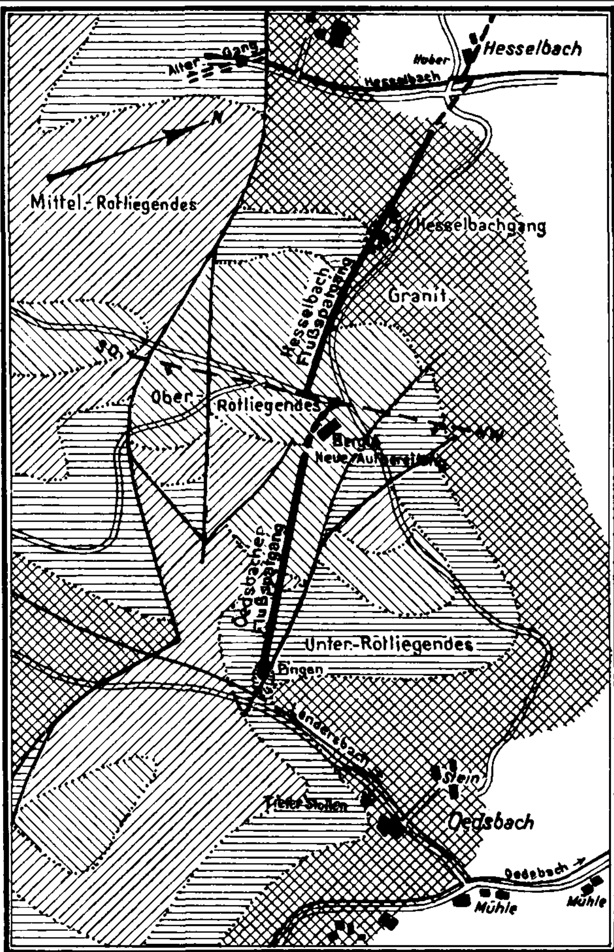
Bild 65. Flußspatvorkommen von Oedsbach-Hesselbach bei Oberkirch, Deutschland
