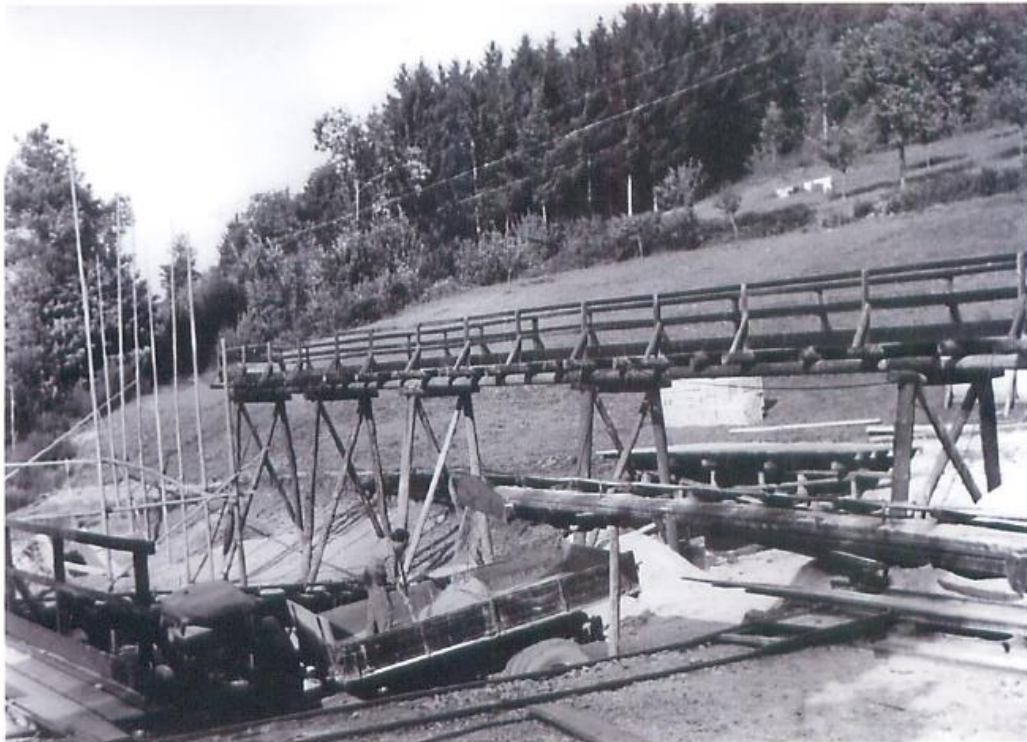
Verladebrücken, mit Lkw zum Bahnhof Oberkirch
